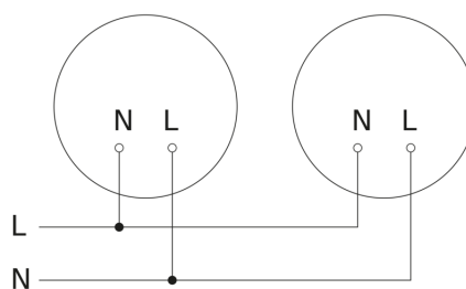
Diagrama electrónico interconexión maestro-maestro
